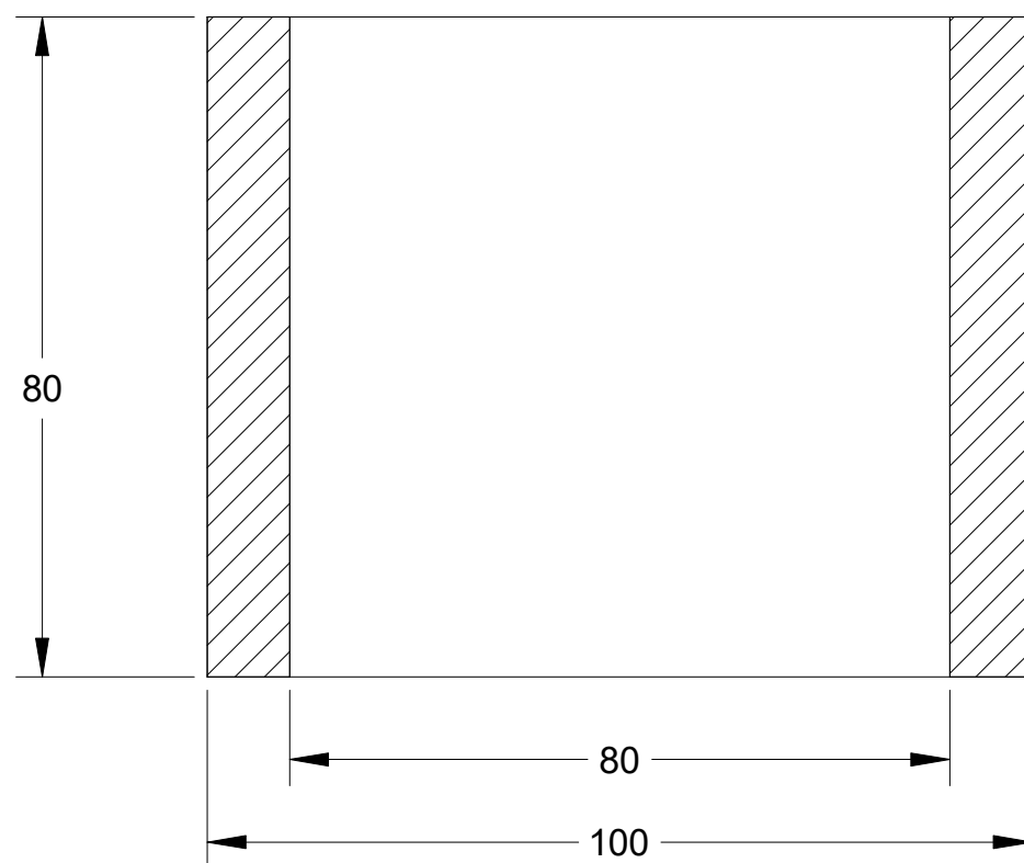
Opzetstuk beton 100x100cm
